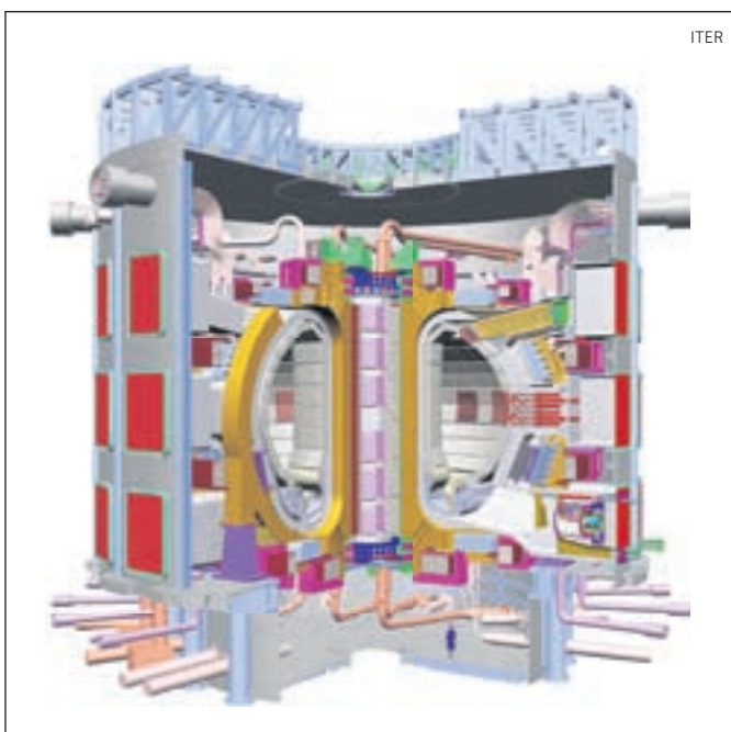
ITER-kooreaktorin suunnitelmapiirros.
